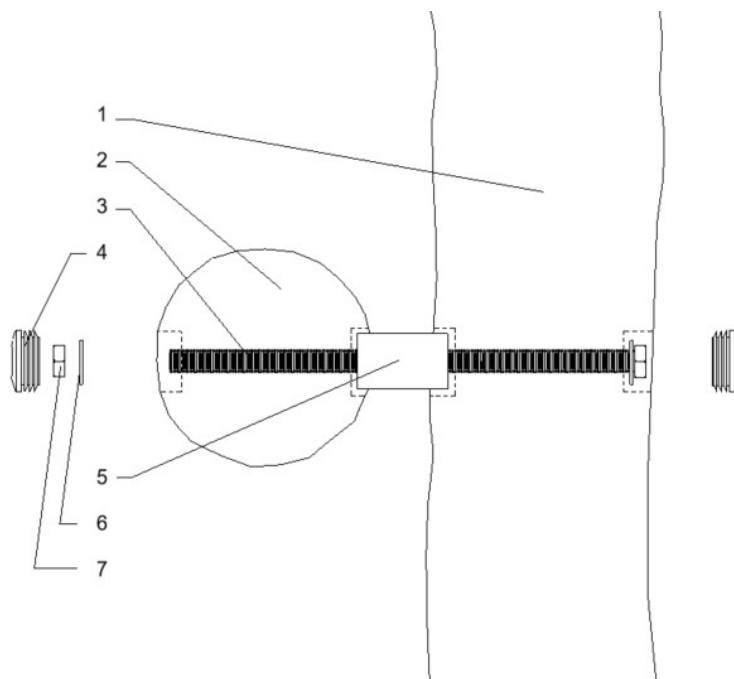
Princip Snitt
