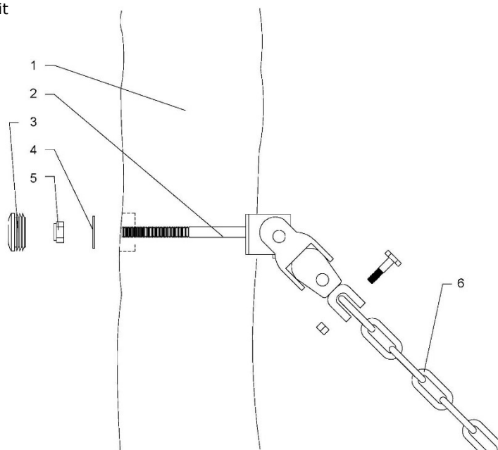
Princip Snit
