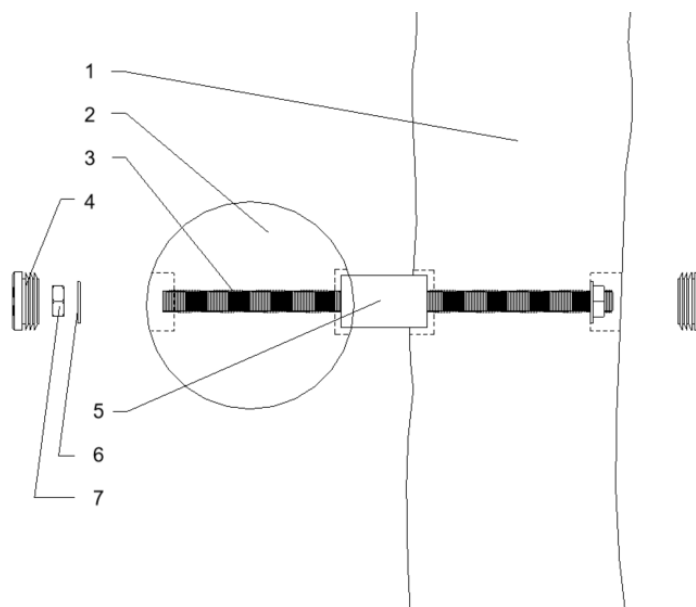
Princip Snit
