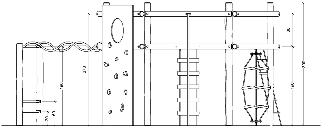
Opstalt front
